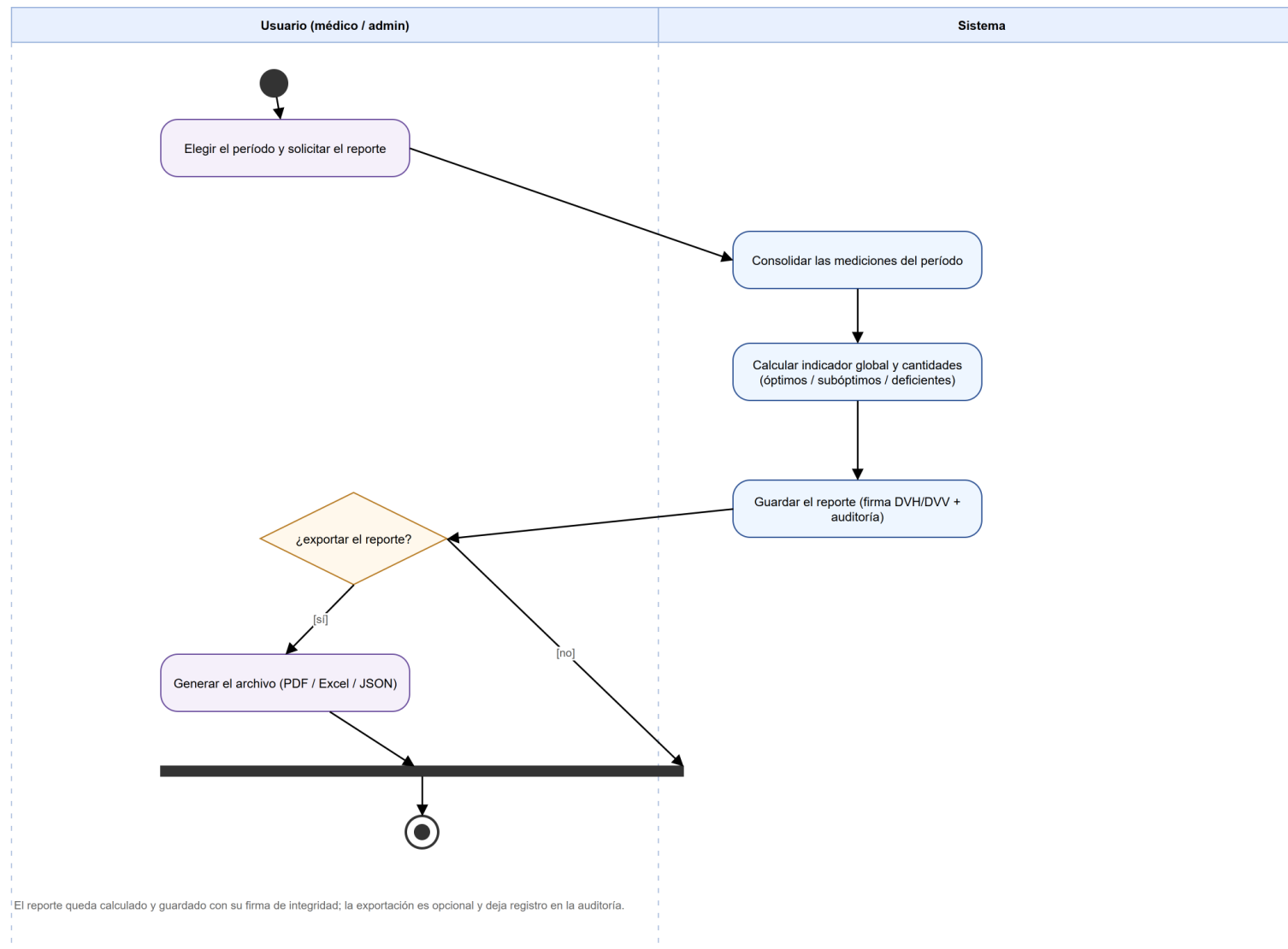
P05 — Diagrama de actividad: generación de reportes estadísticos de eficacia.
