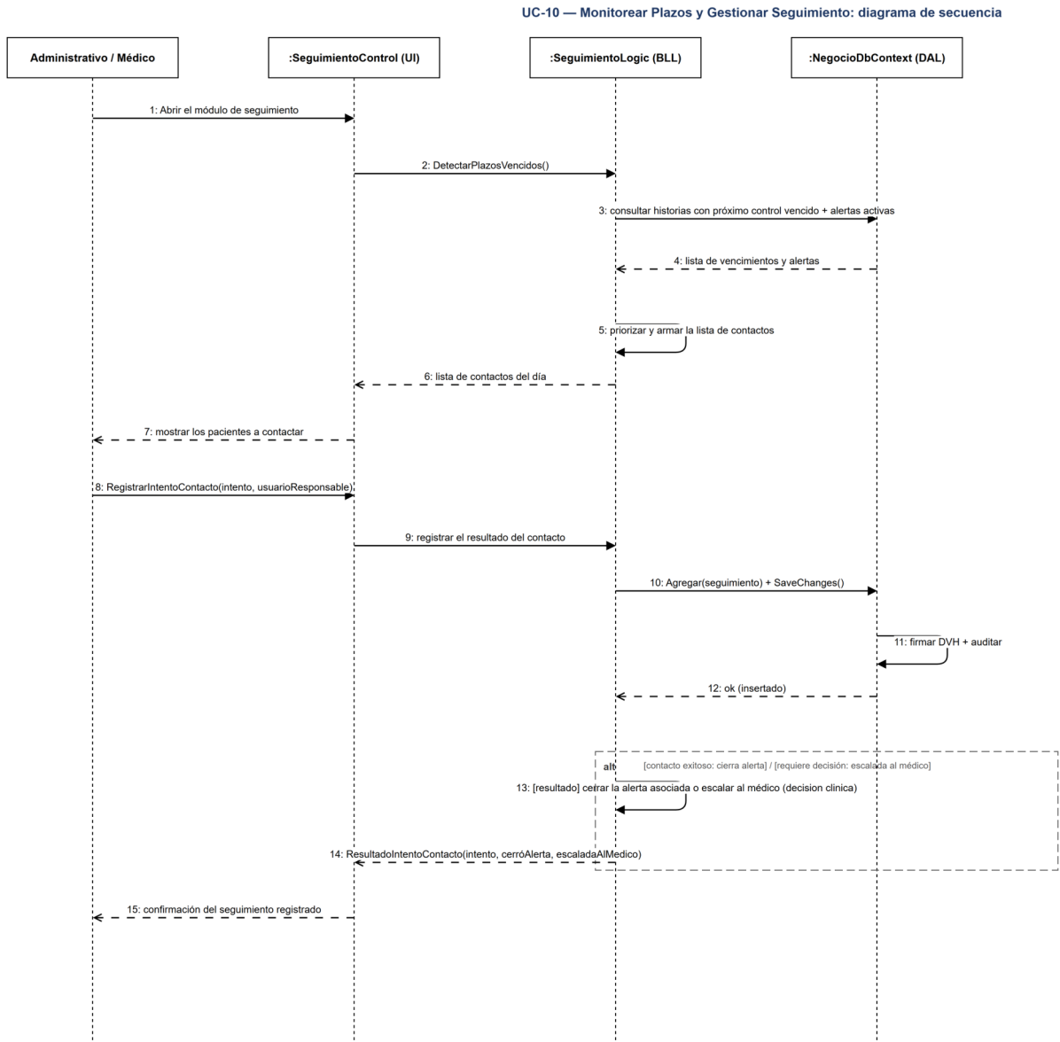
UC-10 — Diagrama de secuencia.
