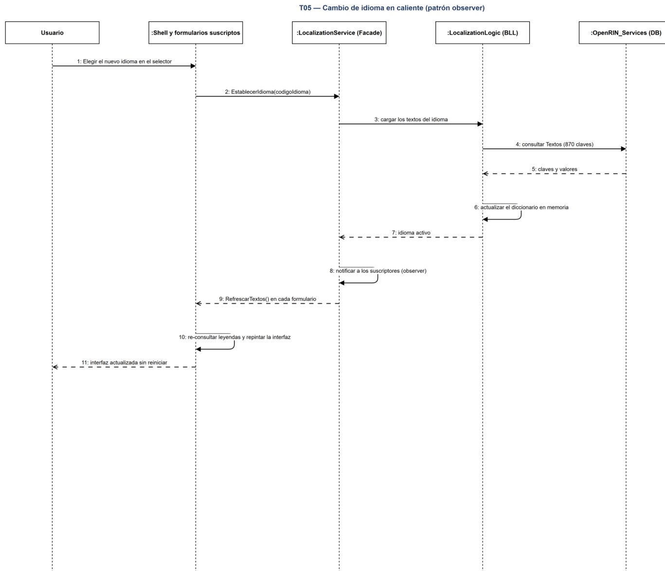
T05 — Secuencia: cambio de idioma en caliente con notificación a los suscriptores (Observer).
