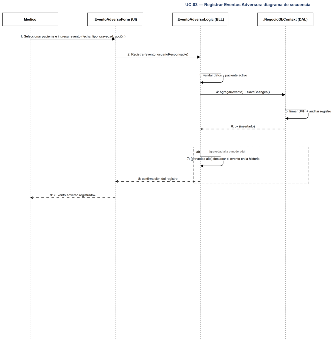
UC-03 — Diagrama de secuencia (registro con destacado).
