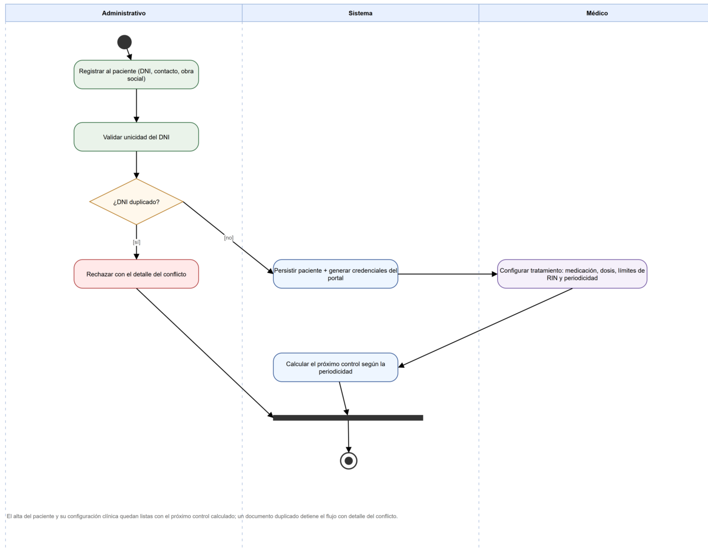
P02 — Diagrama de actividad: configuración de la historia clínica y los parámetros del paciente.
