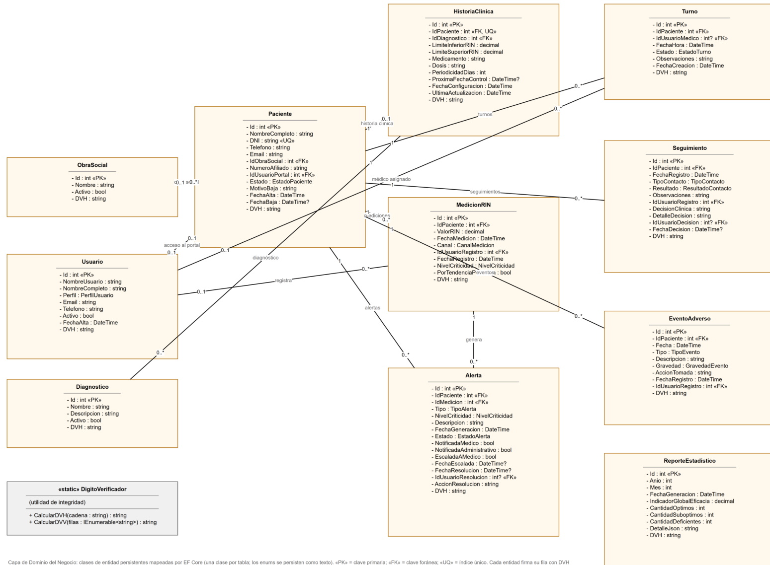
Diagrama de clases — Capa de Dominio del Negocio: entidades persistentes y sus asociaciones (con multiplicidades).
