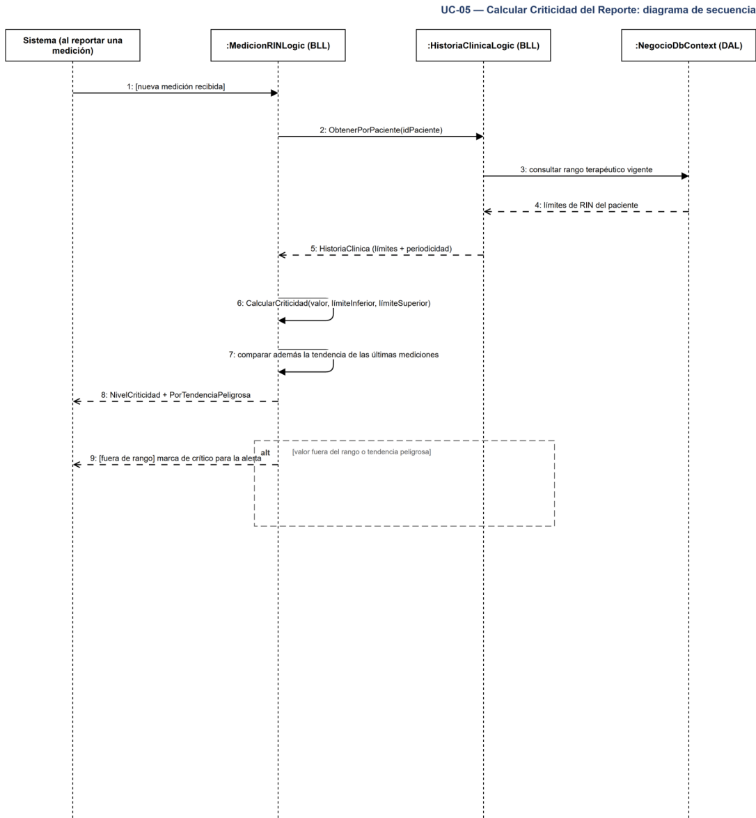
UC-05 — Diagrama de secuencia.
