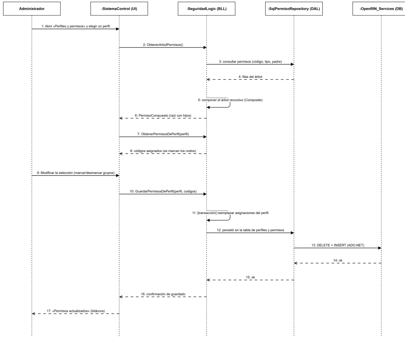
T04 — Secuencia: carga del árbol composite, asignación y persistencia transaccional del perfil.
