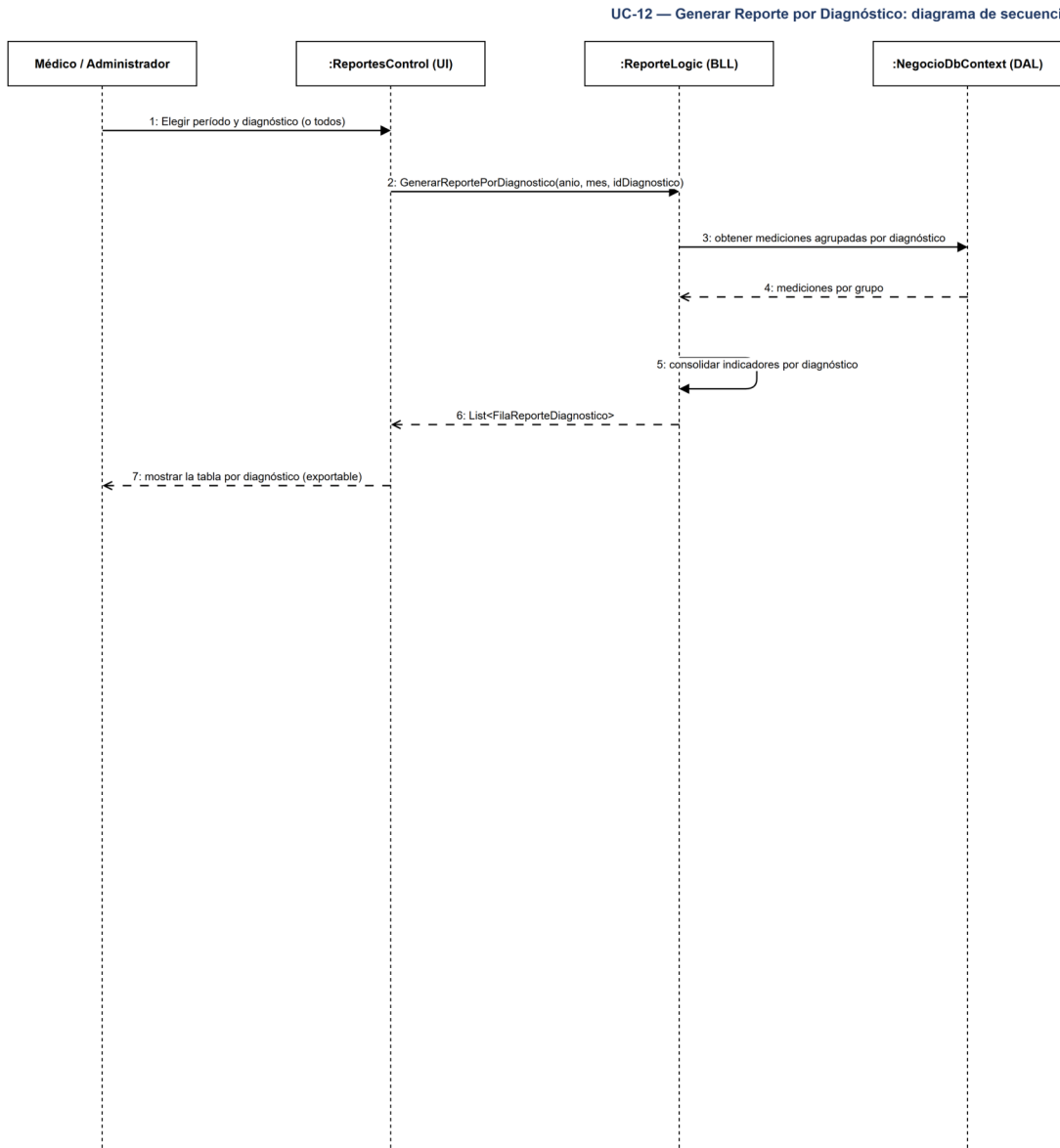
UC-12 — Diagrama de secuencia.
