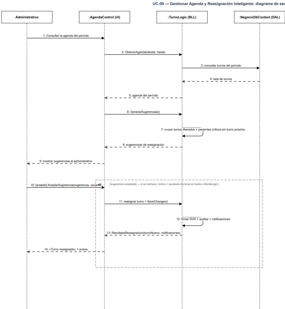
UC-09 — Diagrama de secuencia.
