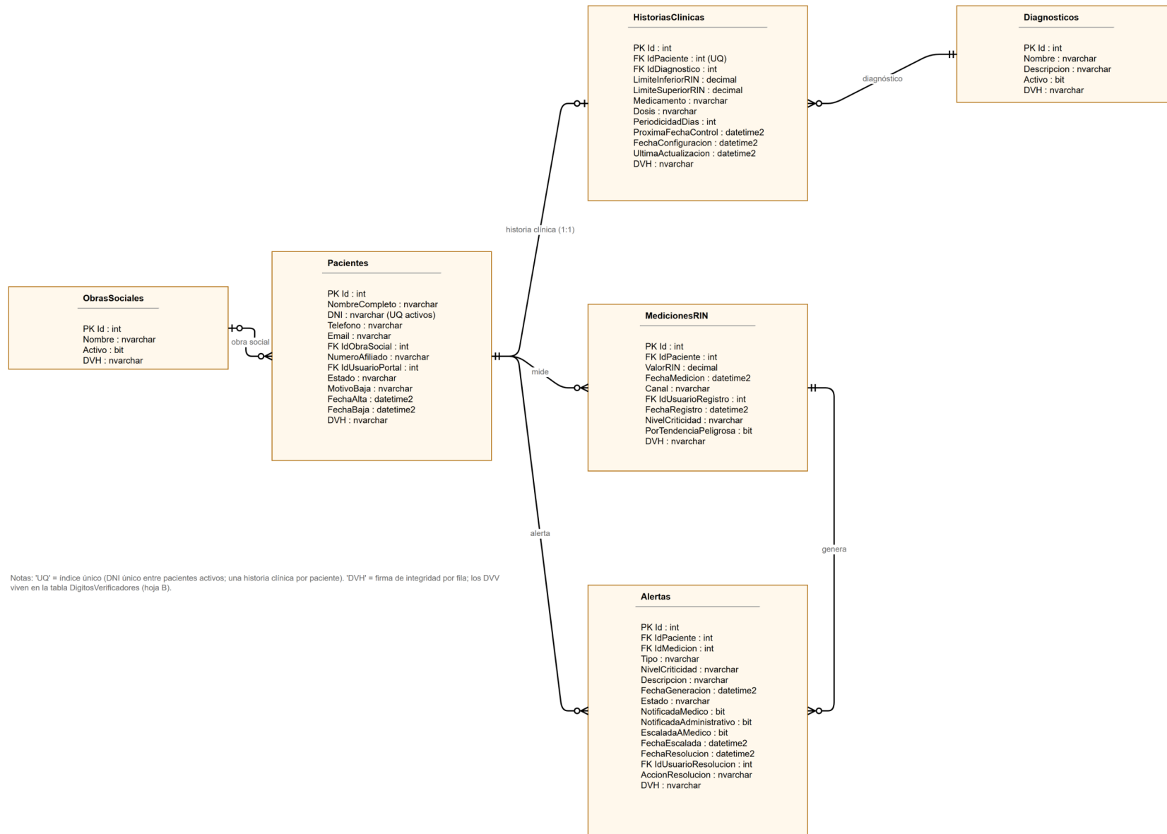
DER (hoja A) — Núcleo clínico: pacientes, historias clínicas, mediciones de RIN y alertas.
