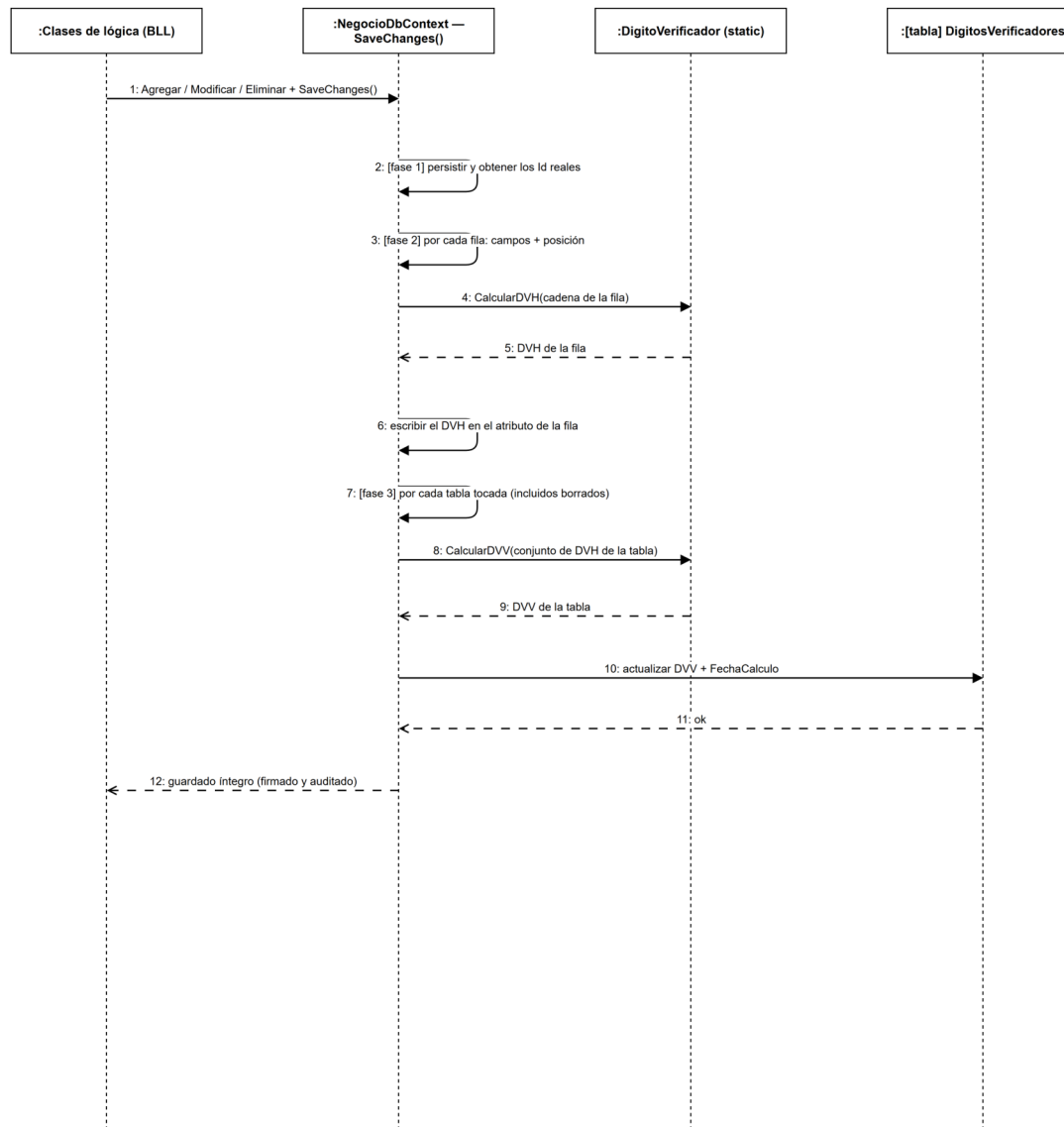
T08 — Secuencia: firma DVH/DVV en el punto único de guardado (3 fases).
