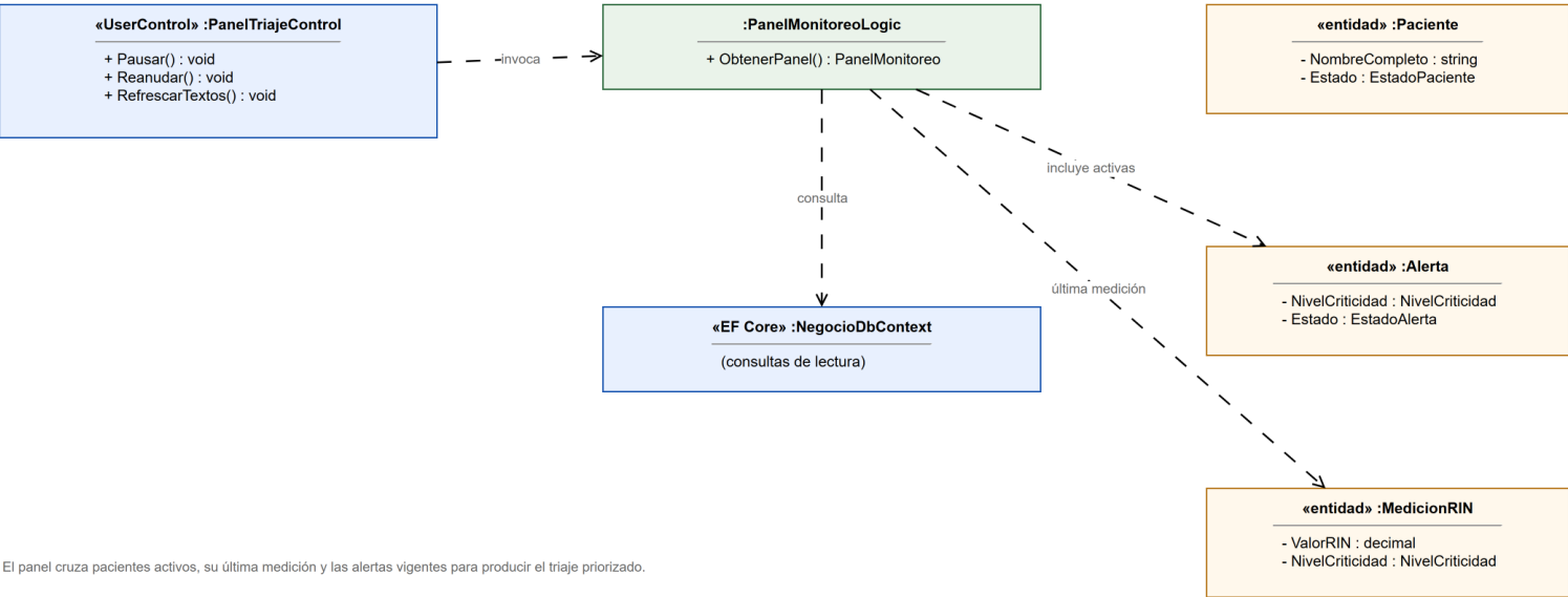
UC-06 — Clases afectadas.
