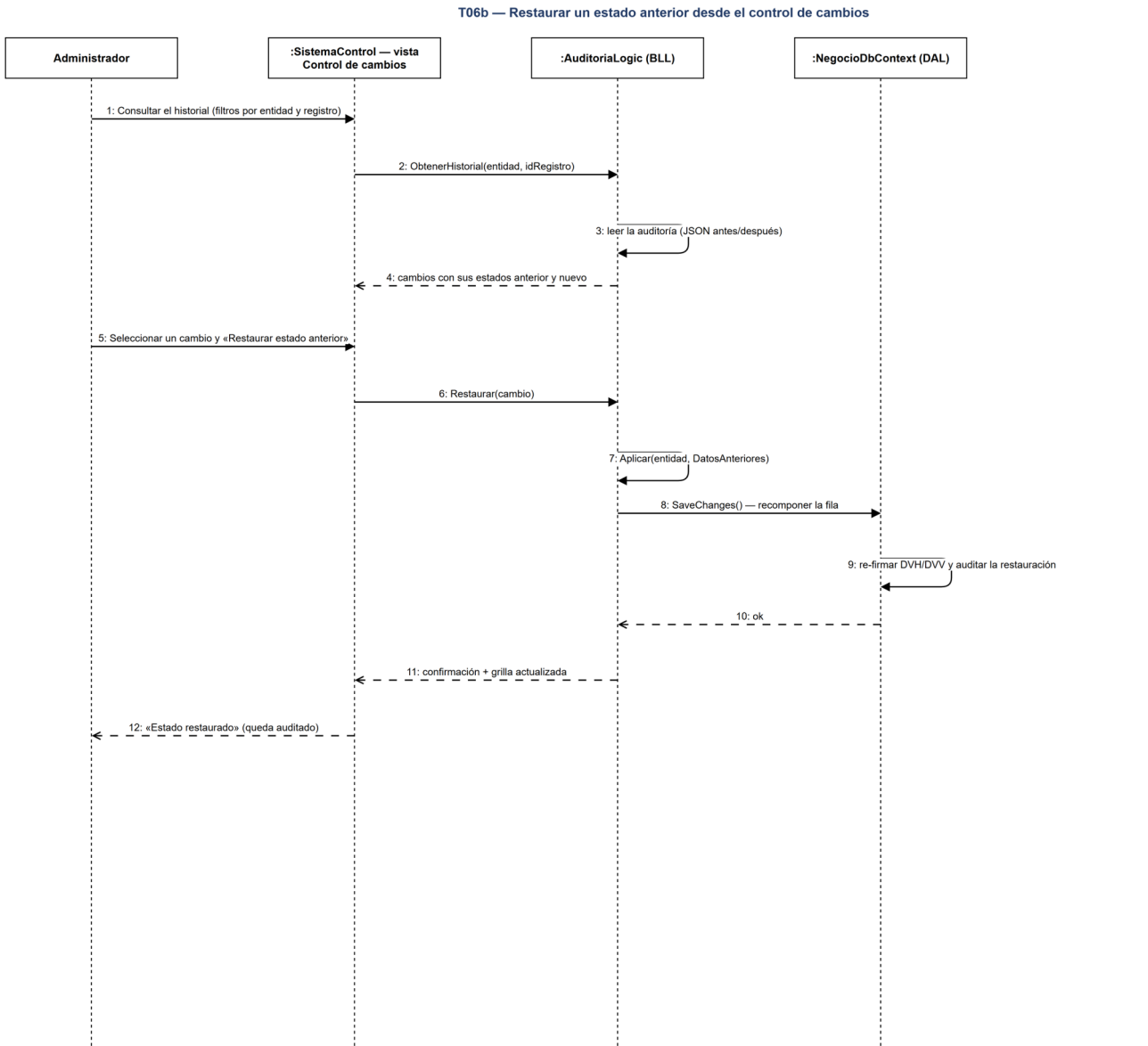
T06b — Secuencia: restauración de un estado anterior con re-firma de integridad y auditoría.
