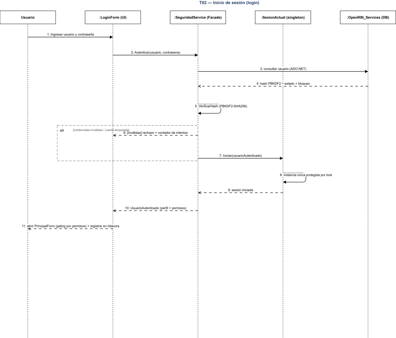
T02 — Secuencia: inicio de sesión con la sesión única (Singleton) y el gating de permisos.
