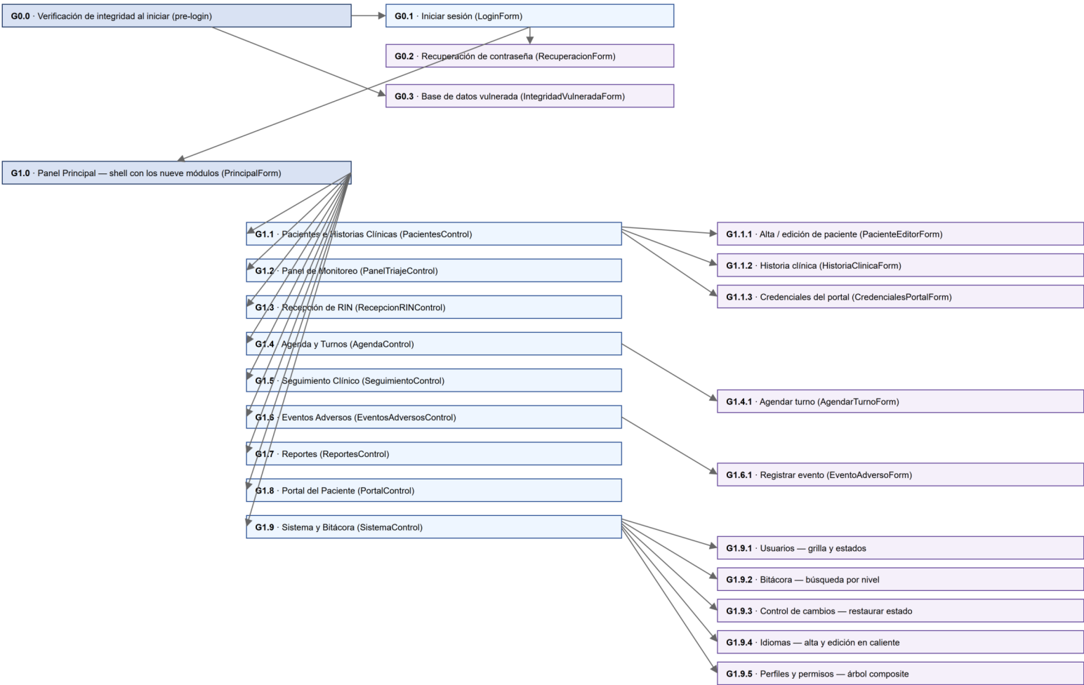
OpenRIN — Mapa de navegación de menús (GUIs con código jerárquico)
