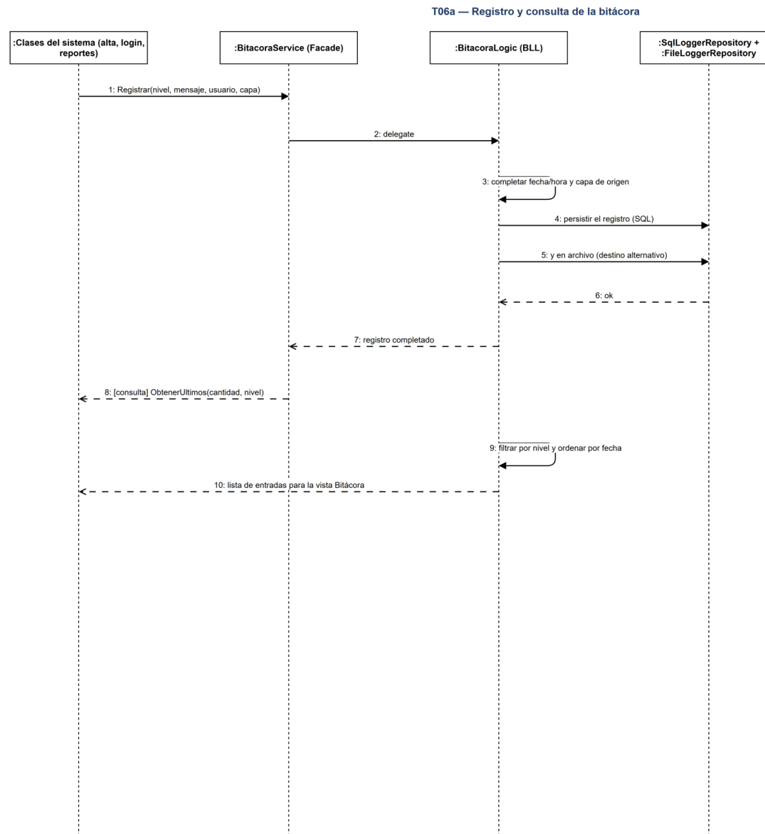
T06a — Secuencia: registro de una entrada en la bitácora (doble persistencia) y su consulta.
