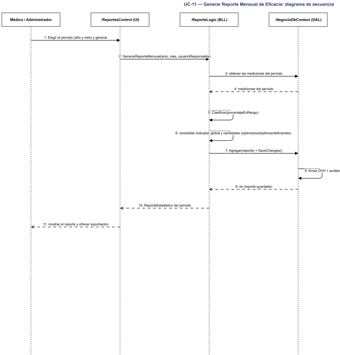
UC-11 — Diagrama de secuencia.
