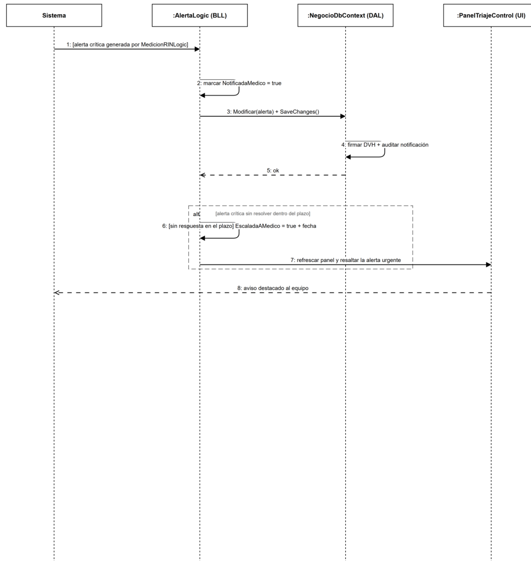
UC-07 — Diagrama de secuencia.
