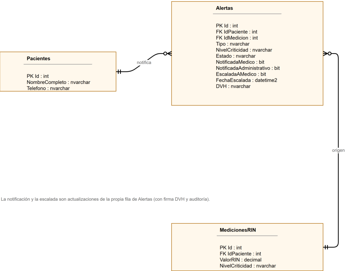
UC-07 — Entidades afectadas (DER parcial).
