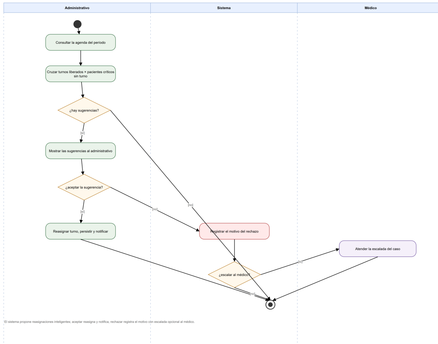
P03 — Diagrama de actividad: optimización de la agenda médica con reasignación.
