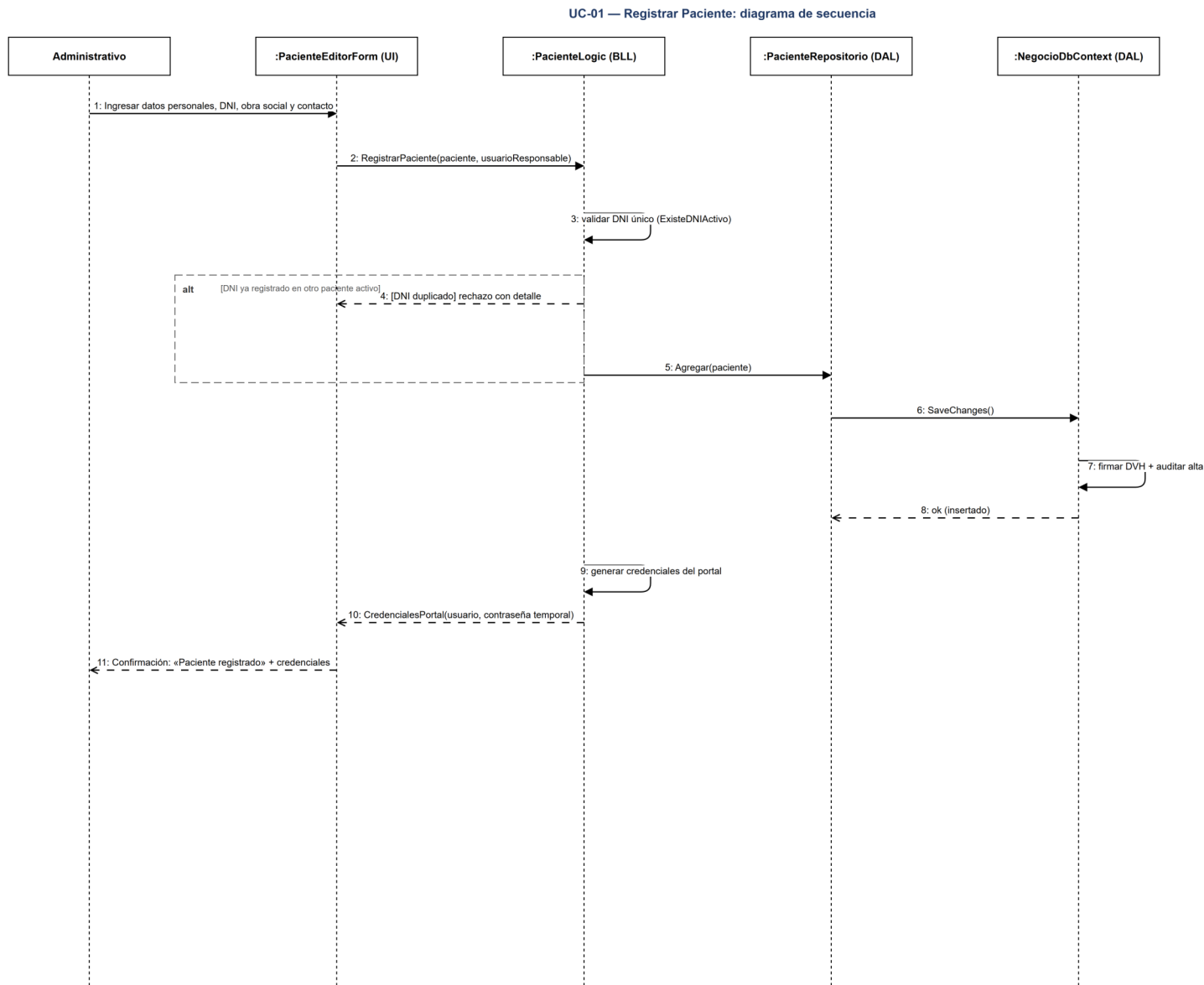
UC-01 — Diagrama de secuencia (alta con validación de DNI).
