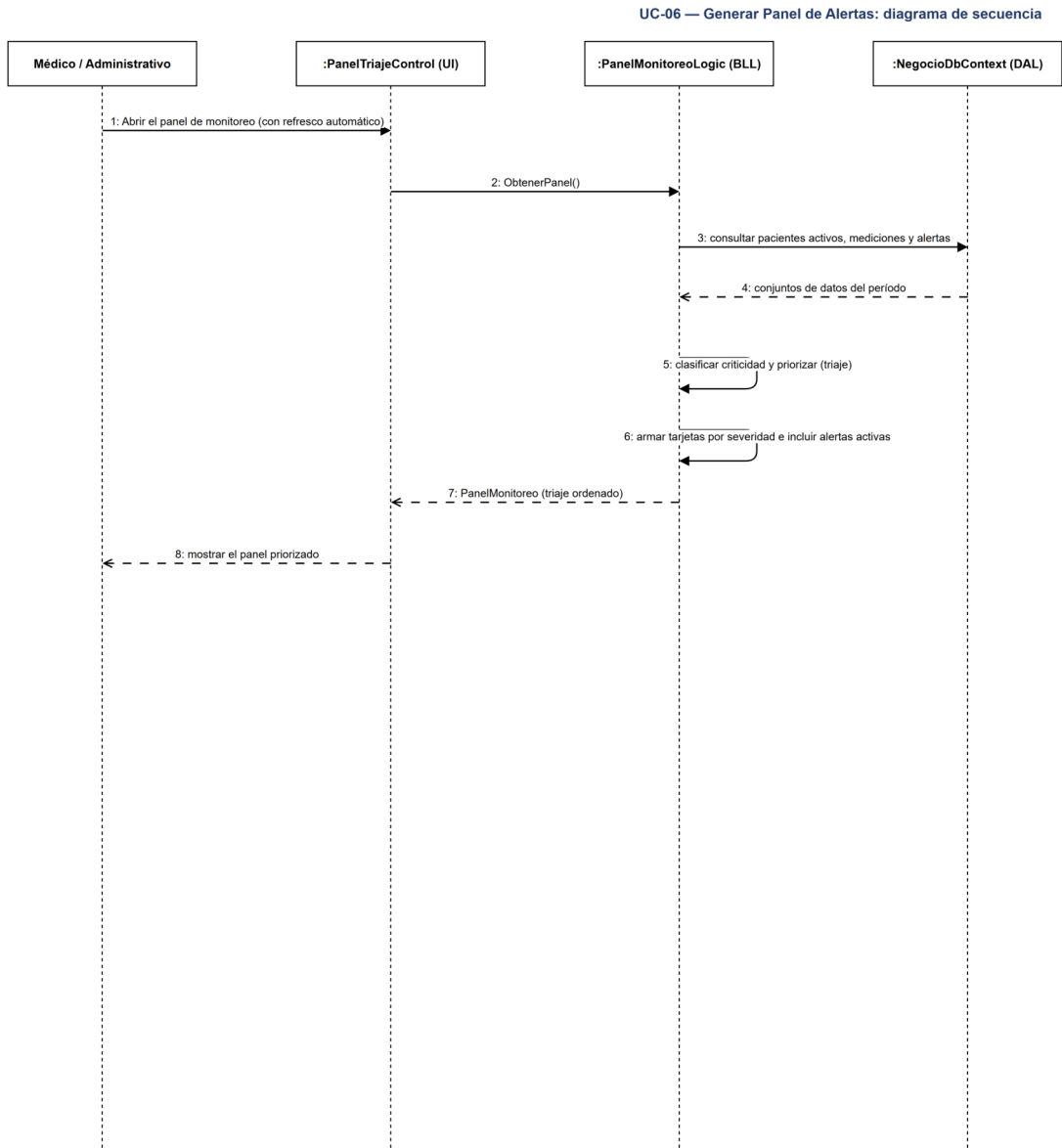
UC-06 — Diagrama de secuencia.
