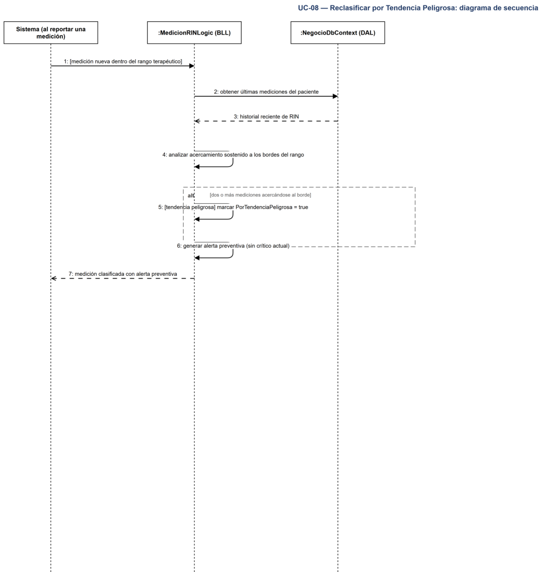
UC-08 — Diagrama de secuencia.
