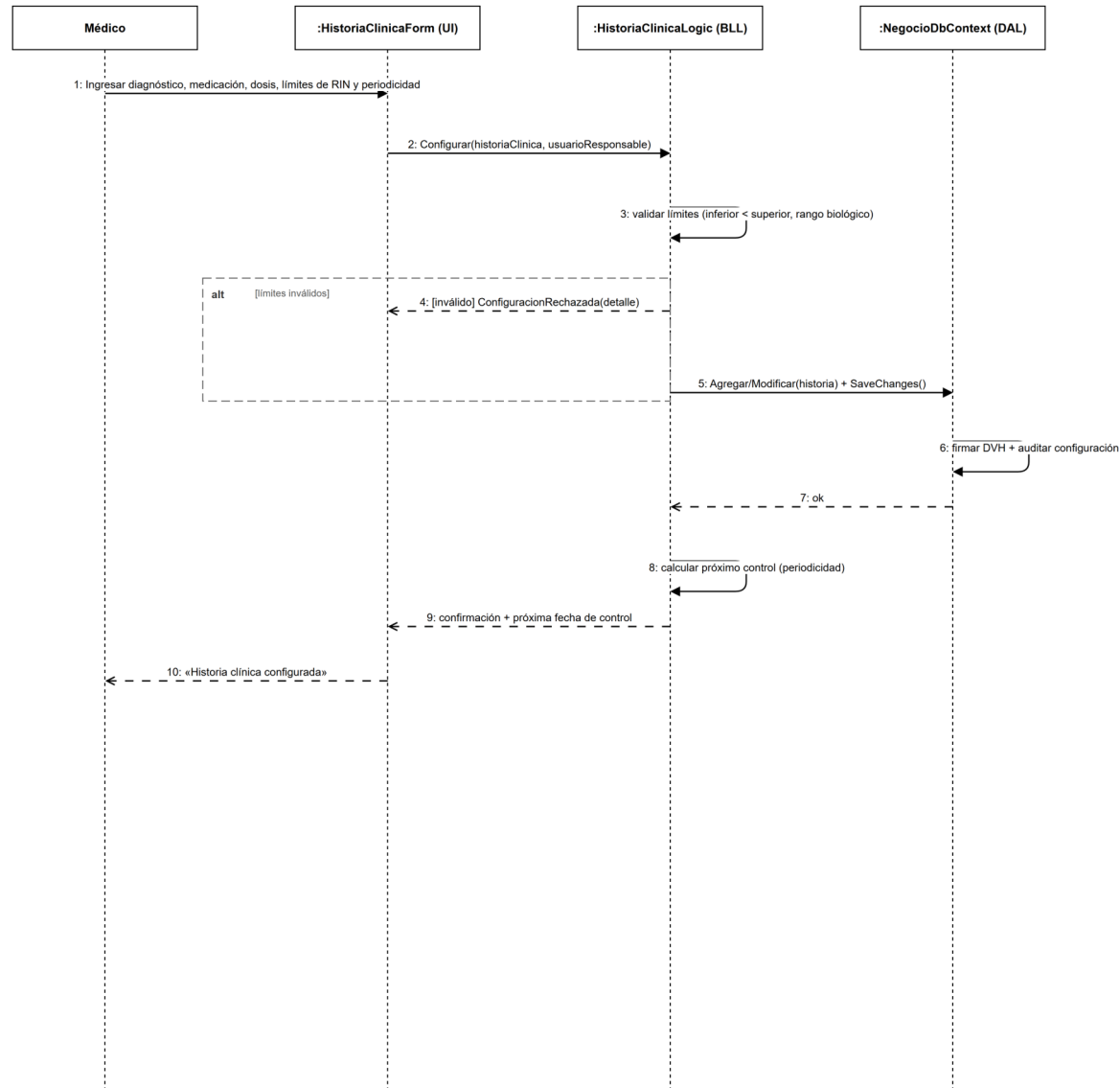
UC-02 — Diagrama de secuencia (configuración y próximo control).
