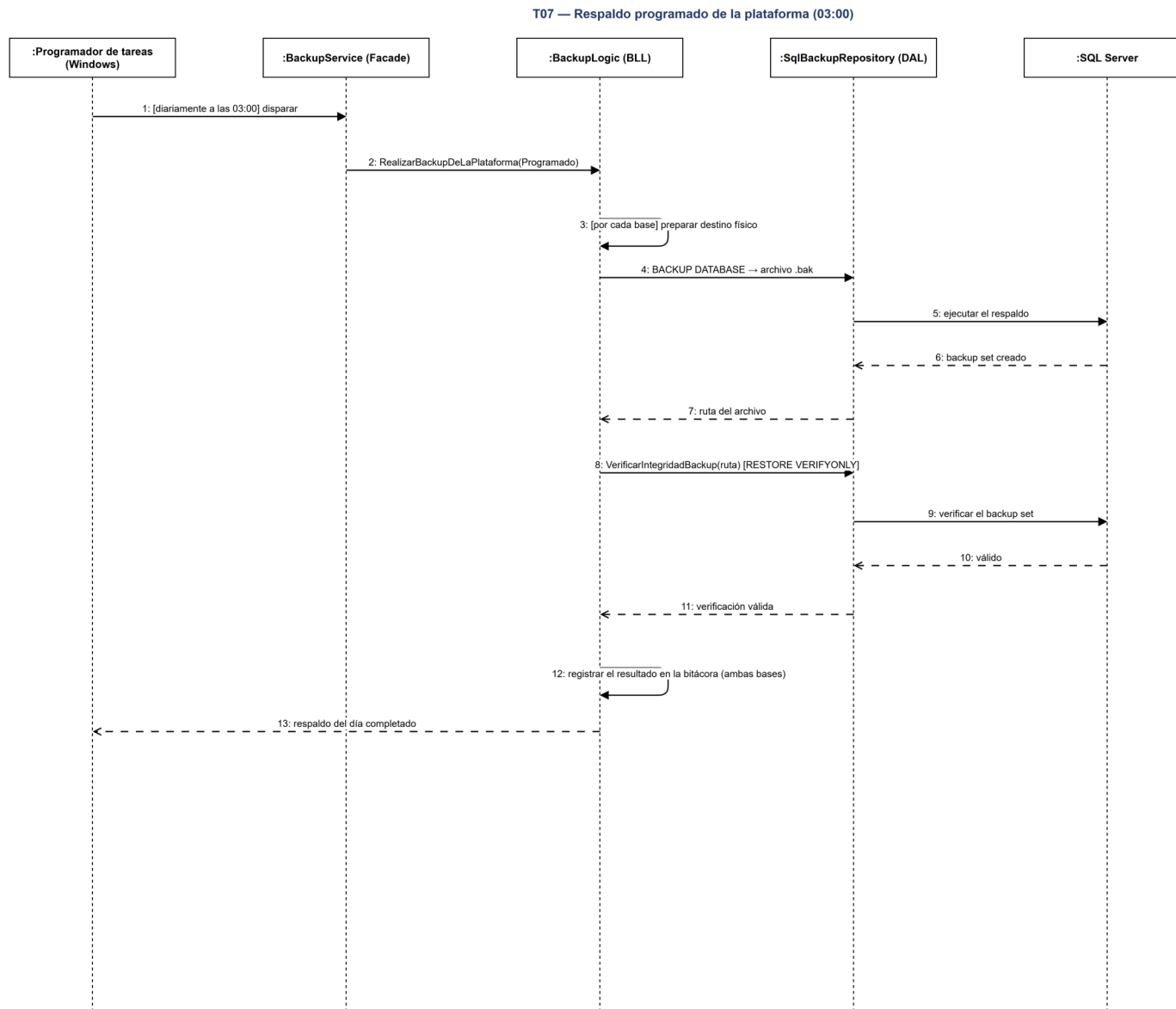
T07 — Secuencia: respaldo programado de la plataforma (03:00) con verificación de integridad de cada copia.
