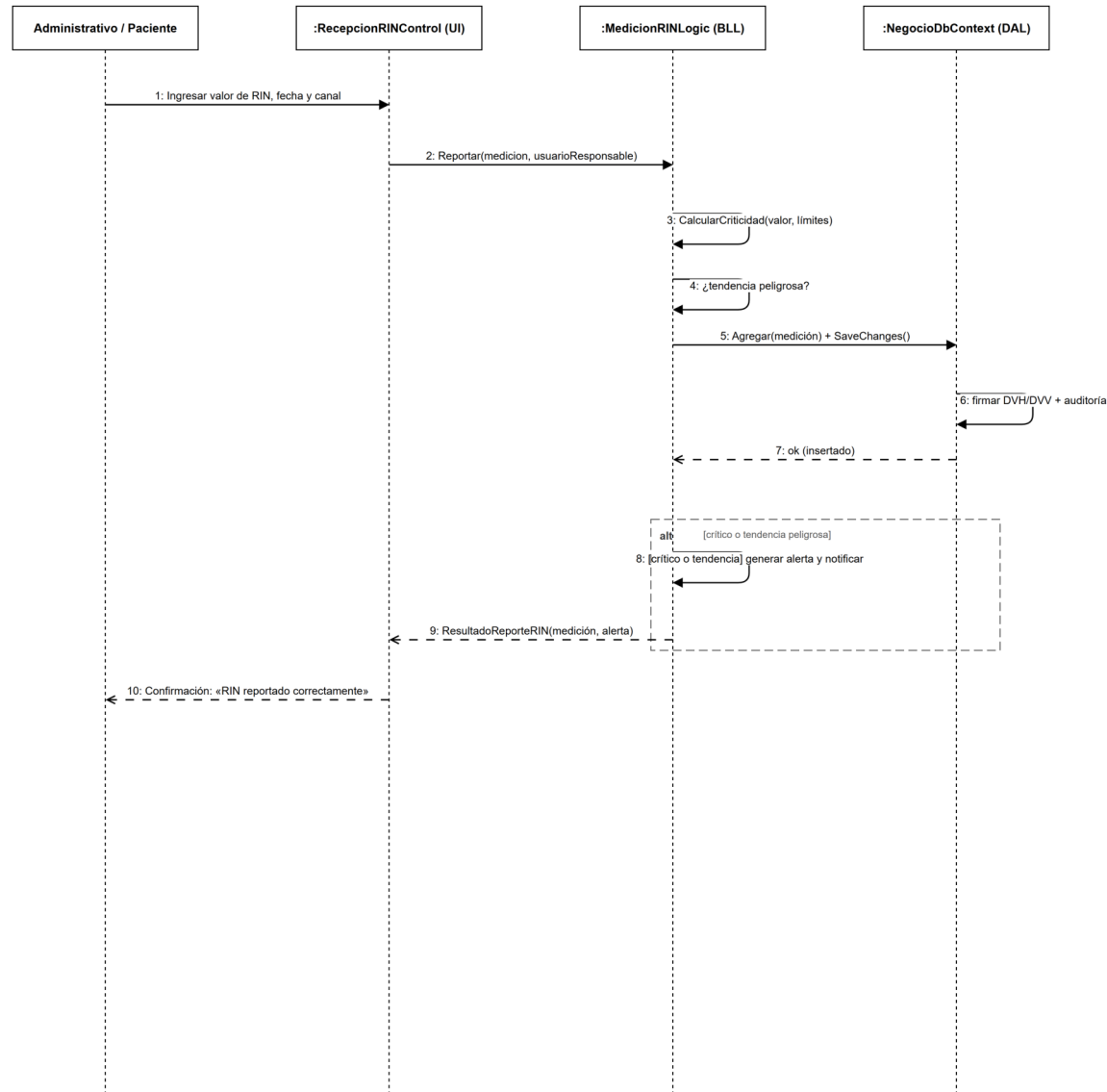
UC-04 — Diagrama de secuencia: flujo normal con generación de alerta (alt).
