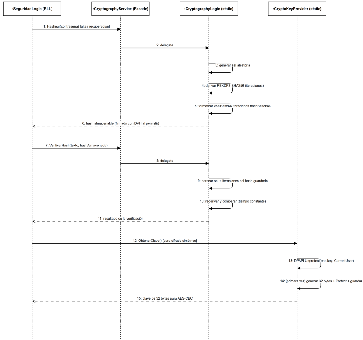
T03 — Secuencia: hasheo/verificación PBKDF2 y la clave protegida por DPAPI.
